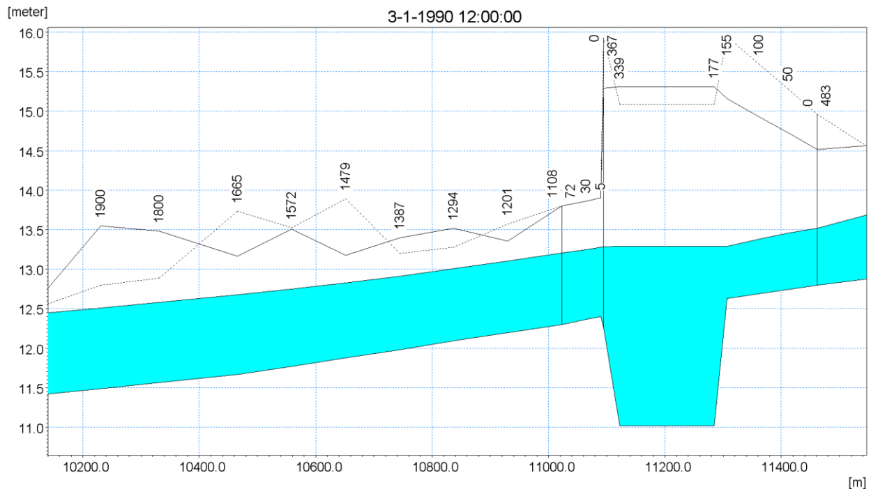
Figur 3-8. Længdeprofil af stryget mellem Holme Kanal og Holme Å ved scenarie A. Vandspejlskoten svarer til en årsmiddelvandføring.
